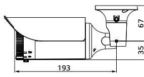
[ LNU3110R / LNU3210R _ Side / Rear ]
